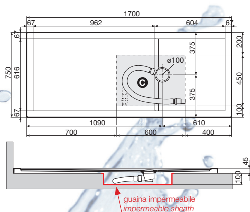
Luna Plus 170x75 - h 4,5 cm
