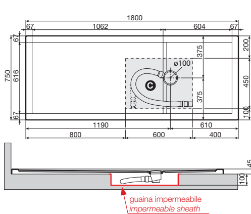
Luna Plus 180x75 - h 4,5 cm
