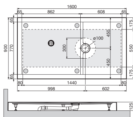
Luna Plus 160x90 - h 12,5 cm
