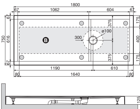
Luna Plus 180x75 - h 12,5 cm
