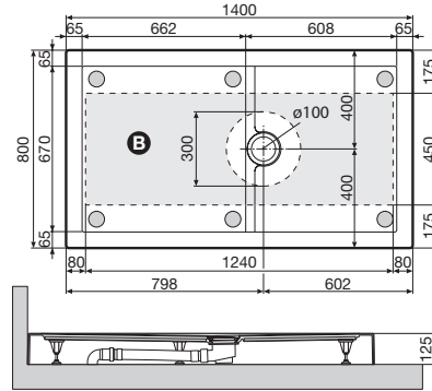
Luna Plus 140x80 - h 12,5 cm
