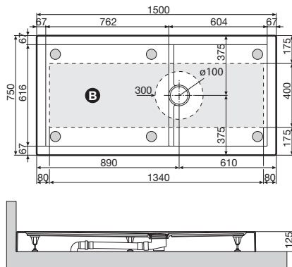
Luna Plus 150x75 - h 12,5 cm
