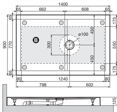
Luna Plus 140x90 - h 12,5 cm
