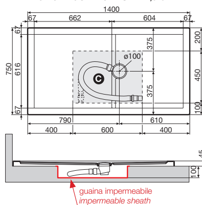
Luna Plus 140x75 - h 4,5 cm
