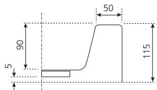
SEZIONE PIATTO DOCCIA bordo h 11,5 cm
