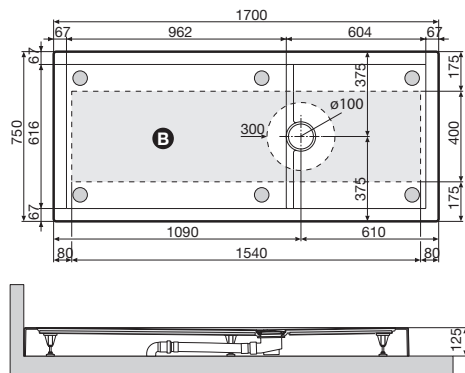
Luna Plus 170x75 - h 12,5 cm
