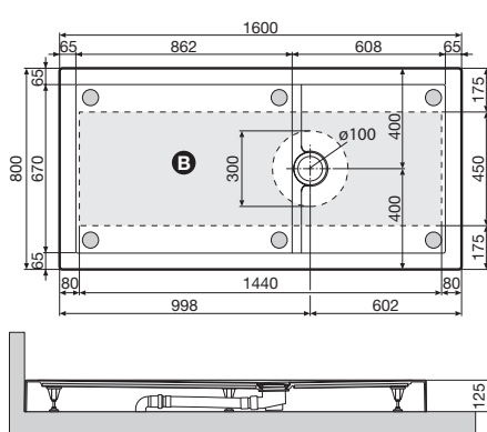
Luna Plus 160x80 - h 12,5 cm
