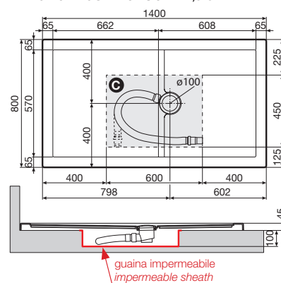
Luna Plus 140x80 - h 4,5 cm
