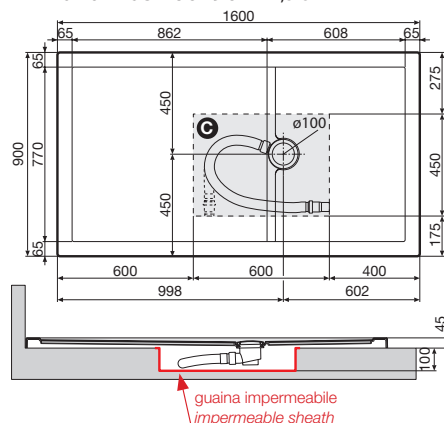
Luna Plus 160x90 - h 4,5 cm
