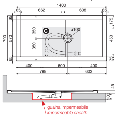
Luna Plus 140x70 - h 4,5 cm
