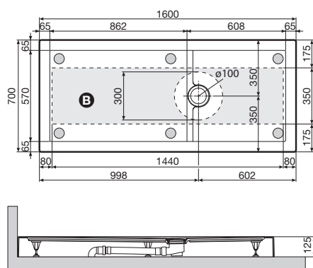
Luna Plus 160x70 - h 12,5 cm
