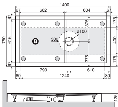
Luna Plus 140x75 - h 12,5 cm
