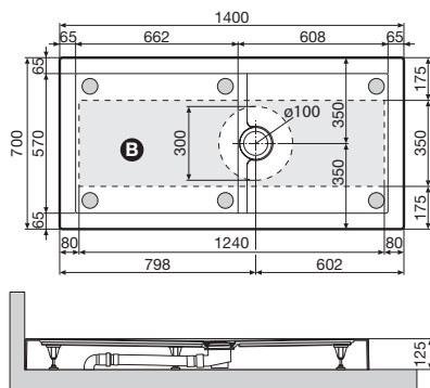
Luna Plus 140x70 - h 12,5 cm
