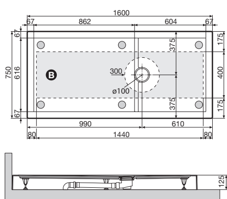
Luna Plus 160x75 - h 12,5 cm
